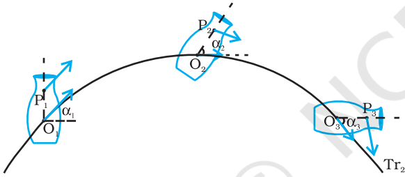
चित्र 6.6(b) दृढ़ पिण्ड की ऐसी गति जो स्थानांतरण और घूर्णी गतियों का संयोजन है
