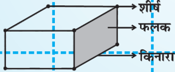
घनाभ
