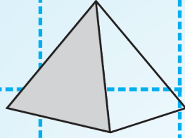
पिरामिड
