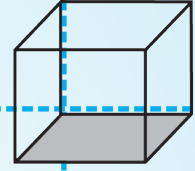
घन
