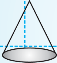
शंकु
