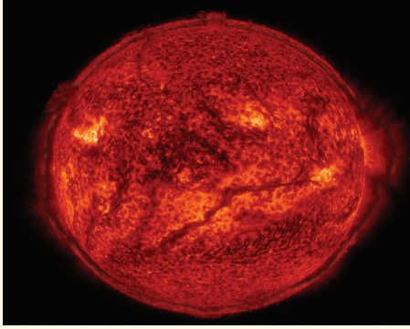
চিত্ৰ ১.৩ : সূৰ্য
