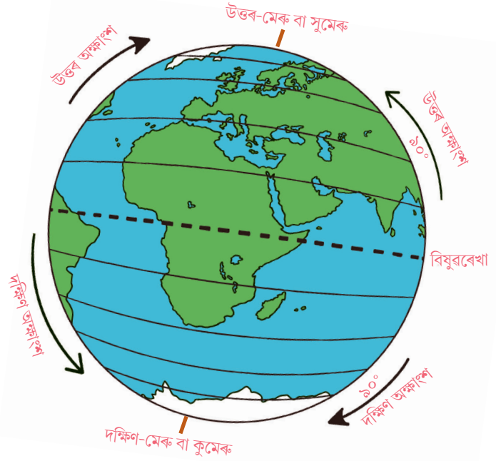
চিত্ৰ ১.৮ : অক্ষৰেখা
