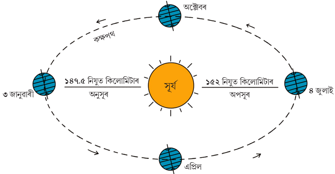
চিত্ৰ ১.১১: অনুসূৰ আৰু অপসূৰ
