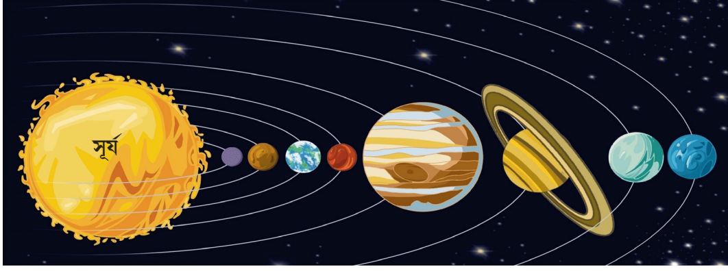
চিত্ৰ ১.২ : সৌৰজগত
