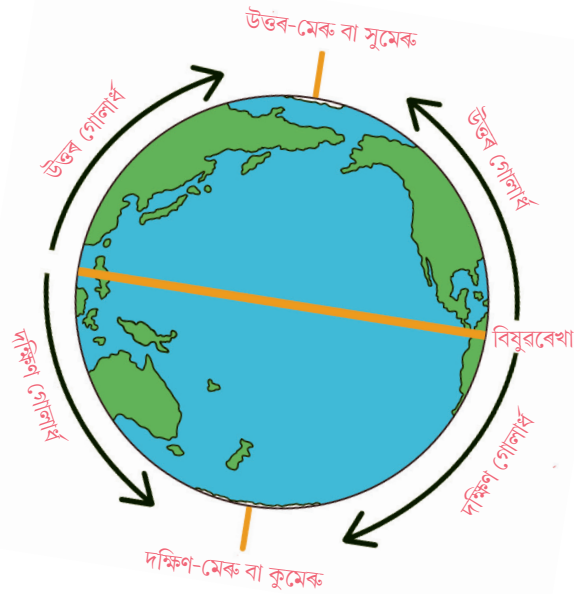
চিত্র ১.৭ : বিষুবৰেখা
