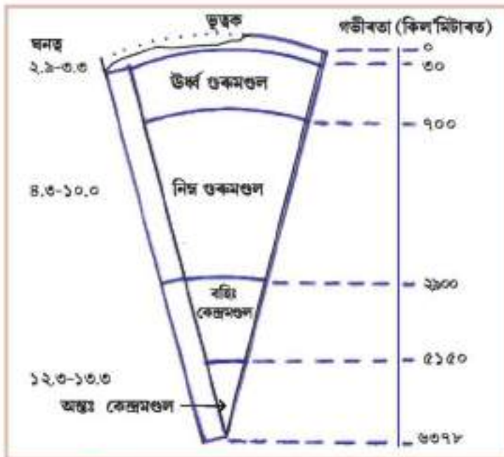
চিত্ৰ : ২.২ পৃথিৱীৰ অভ্যন্তৰভাগৰ স্তৰসমূহ
