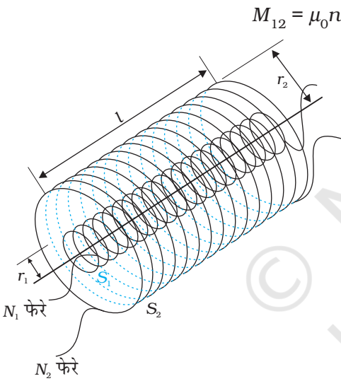
चित्र 6.12 समान लंबाई l की दो समाक्षी दीर्घ परिनालिकाएँ।
