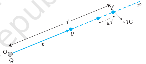
चित्र 2.3 आवेश Q के कारण बिंदु P पर विभव, किसी एकांक धनात्मक परीक्षण आवेश को, आवेश Q ( Q > 0 ) के कारण प्रतिकर्षण बल के विरुद्ध, अनंत से बिंदु P तक लाने में किए गए कार्य के बराबर होता है।
