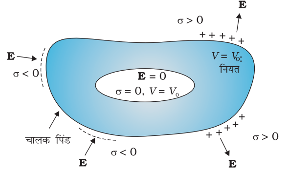
चित्र 2.18 किसी भी चालक की कोटर (गुहा) के भीतर विद्युत क्षेत्र शून्य होता है। चालक का समस्त आवेश कोटर सहित उस चालक के केवल बाह्य पृष्ठ पर ही विद्यमान रहता है (कोटर के भीतर कोई आवेश नहीं रखे गए हैं)।
